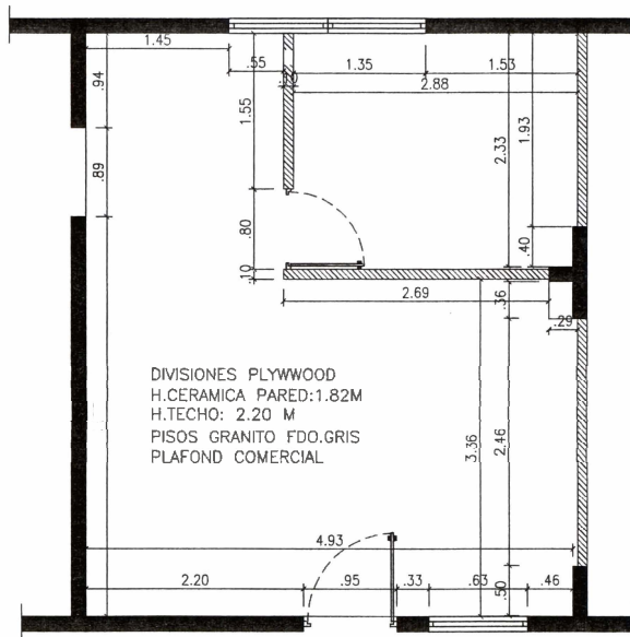
DISPENSARIO MEDICO PLANTA DE LEVANTAMIENTO 1ER NIVEL
