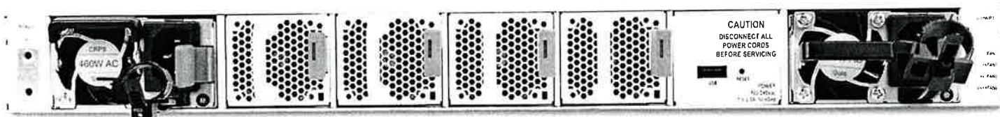
FortiSwitch 1048E — back
