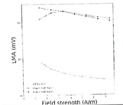
Curva Amplitud de Modulación de Carga de la Muestra 1 para f_c/128
