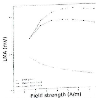
Curva Amplitud de Modulación de Carga de la Muestra 2 para f_c/2
