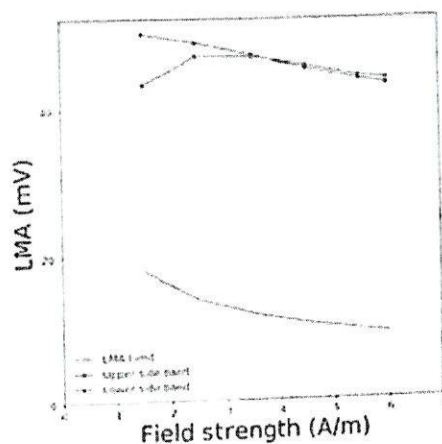
Curva Amplitud de Modulación de Carga de la Muestra 1 para f_c/128
